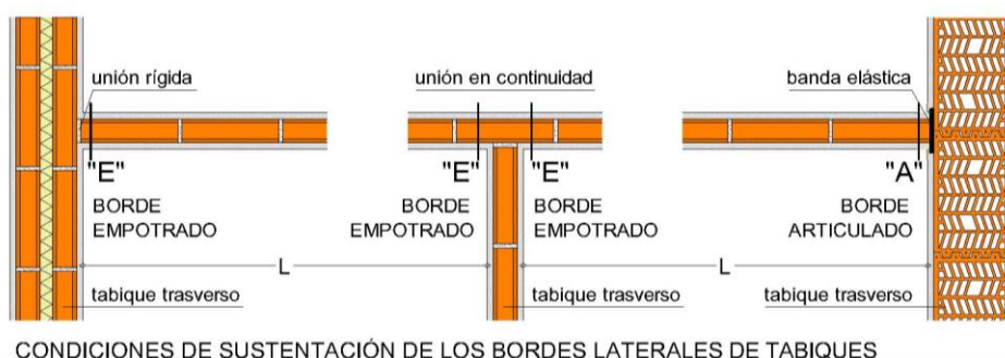
CONDICIONES DE SUSTENTACIÓN DE LOS BORDES LATERALES DE TABIQUES
