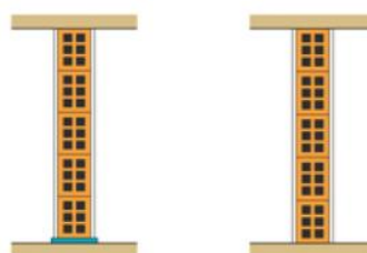
Tabiques con bandas elásticas en la base
